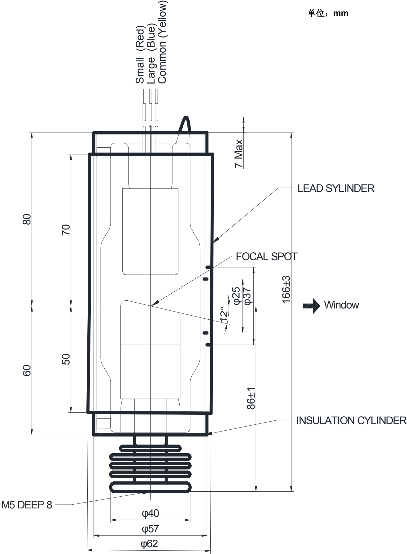
X 射线管外形尺寸图 -XD25-0.6/1.5-125SBR
